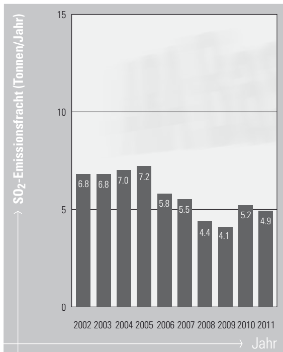
Figur 12 Emissionsfracht an SO 2 im Rauchgas Schlammbehandlung
