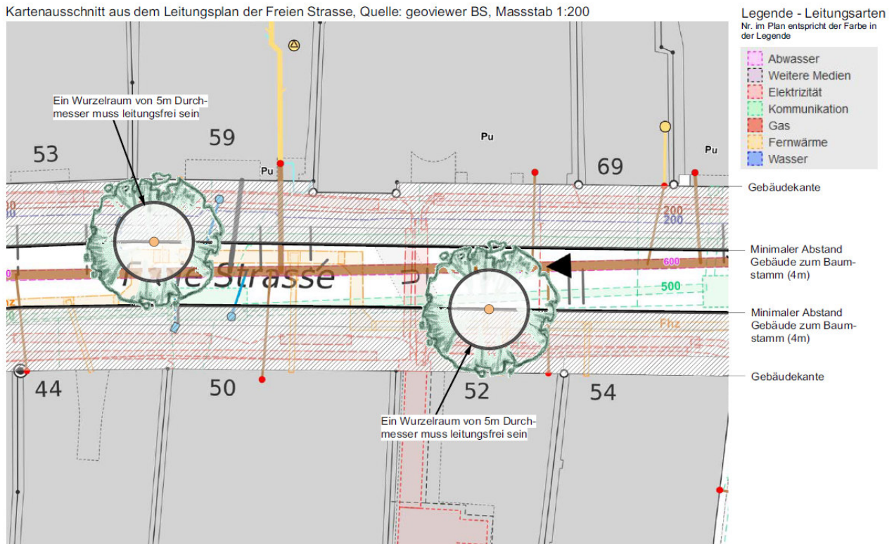
Abbildung 1: Leitungsplan Freie Strasse
